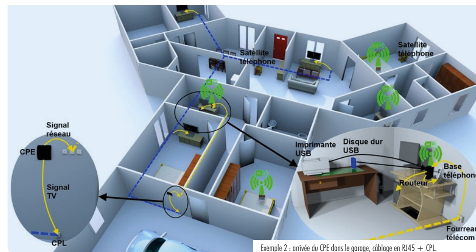
Exemple 2 : arrivée du CPE dans le garage, câblage en RJ45 + CPL.
