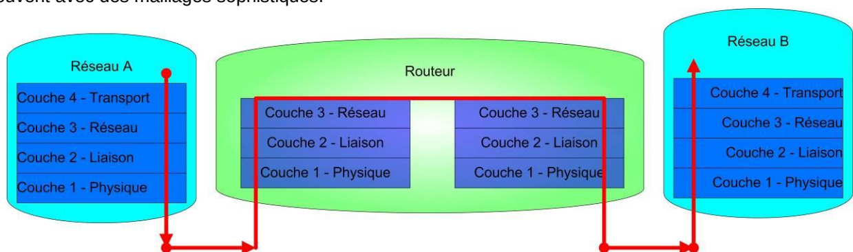
Routeurs - Principes de fonctionnement.
