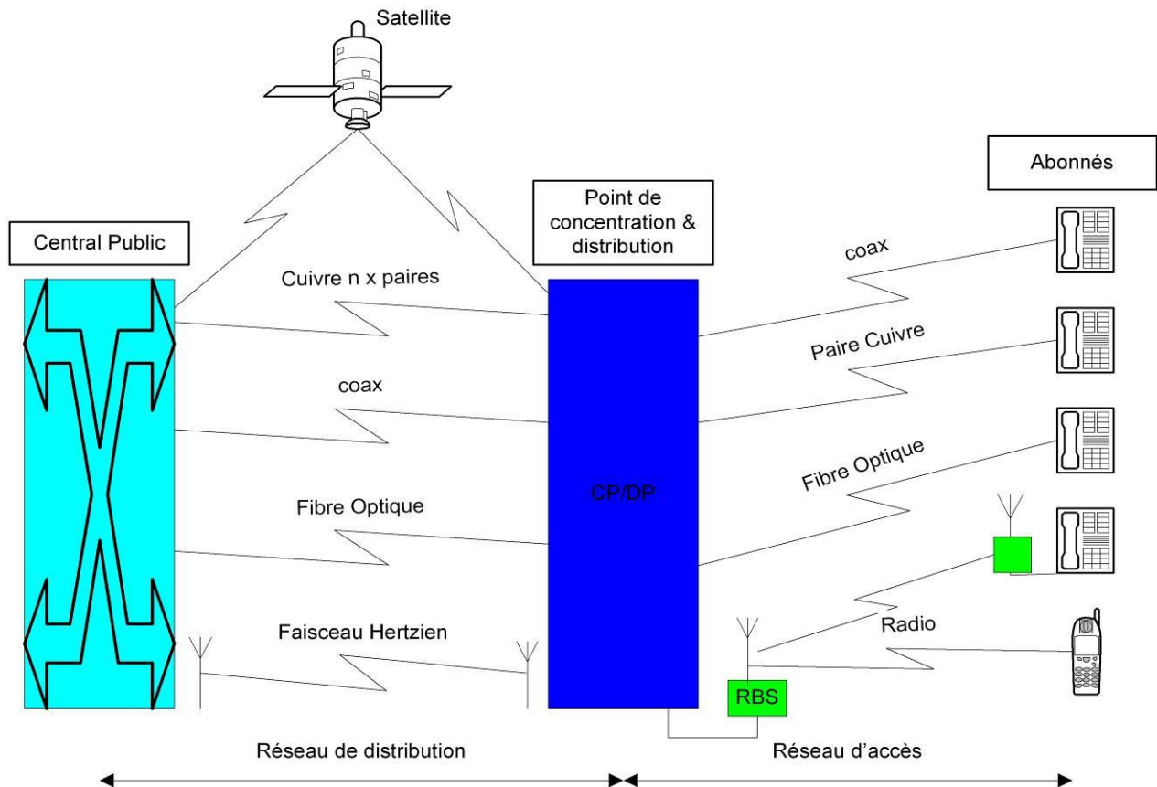
Représentation schématique de la boucle locale
