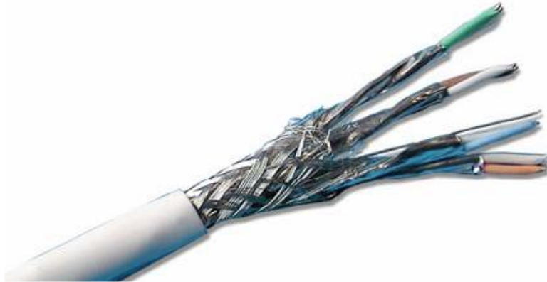
Câble catégorie 7
