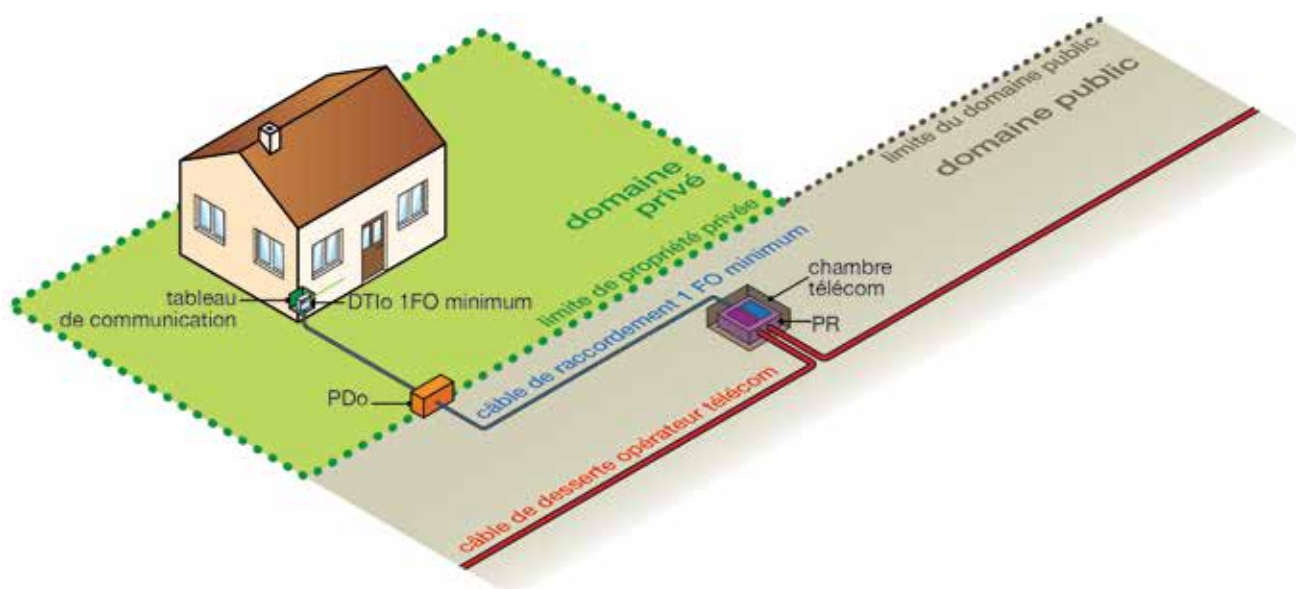
Figure 7 : Maison isolée sur terrain avec raccordement souterrain à un PR distant
