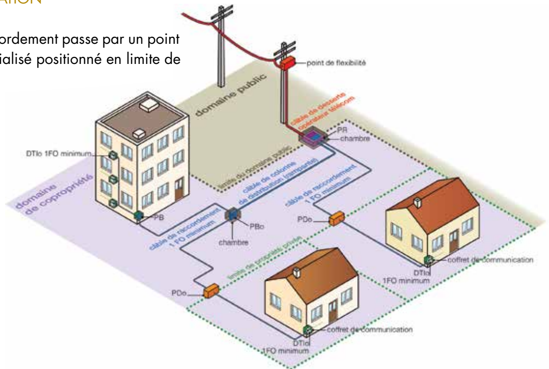
Figure 13 : Lotissement mixte en copropriété avec raccordement souterrain
