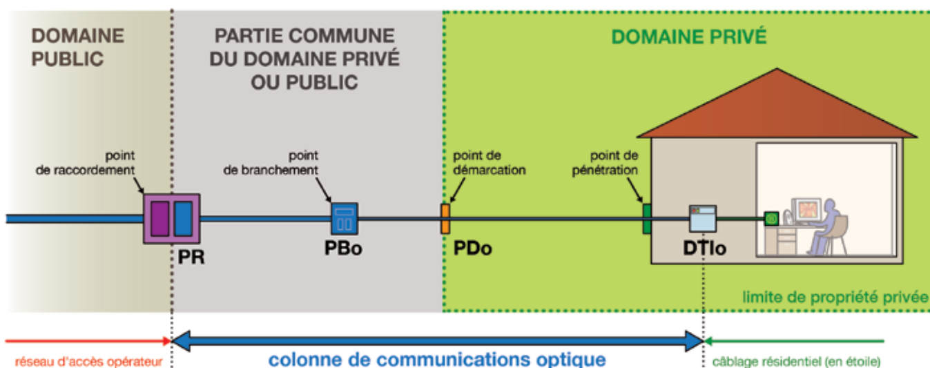
Figure 1 : Synoptique général de la colonne de communication
