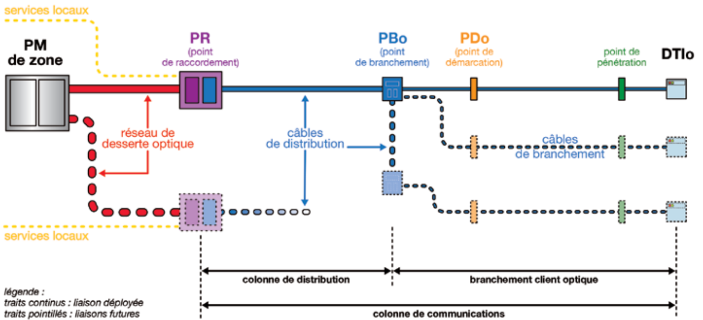
Figure 2 : Synoptique détaillé de la colonne de communication
