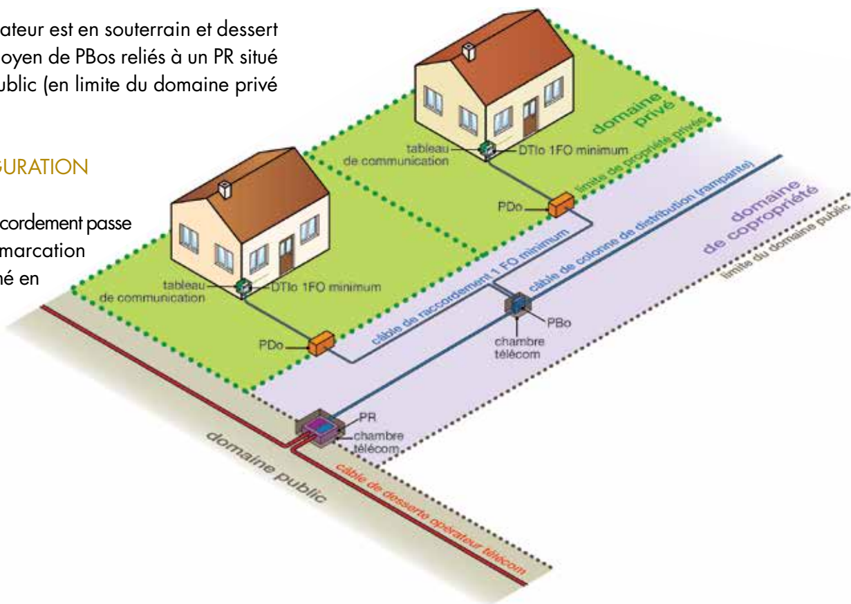
Figure 11 : Maison individuelle en lotissement avec copropriété avec point de démarcation
