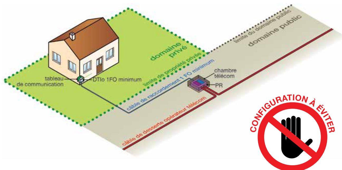
Figure 8 : Maison isolée sur terrain avec raccordement souterrain à un PR distant
