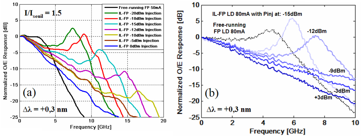
FIGURE 2.25 – Réponse en fréquence en modulation petit-signal du laser Fabry-Perot optiquement injecté : Run1 (a) et Run2 (b) [33]
