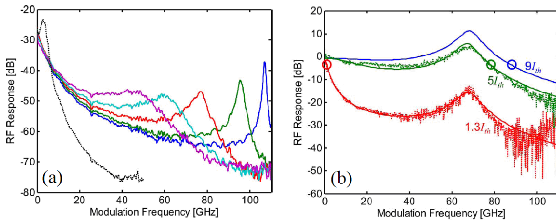
FIGURE 2.26 – Exemples de la réponse en fréquence d'un laser VCSEL injecté pour différents désaccords (a) et pour différents courants de polarisation (b) (d'après K. Lau et al. [28, 29, 30])
