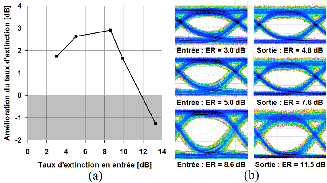
FIGURE 3.28 – Amélioration du taux d’extinction par le R-EAM-SOA (a) et illustration par les diagrammes de l’oeil à 10 Gb/s (b) (ER : Extinction Ratio)
