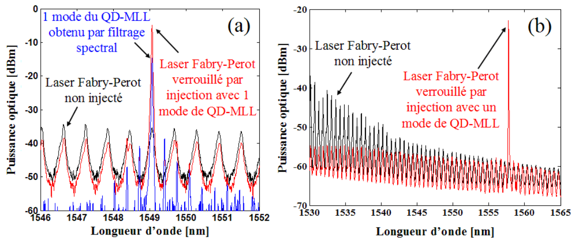
FIGURE 5.13 – Spectres optiques du laser Fabry-Perot verrouillé par injection optique avec un mode de QD-MLL sur une plage de 6 nm (a) et de 35 nm (bande C) (b)
