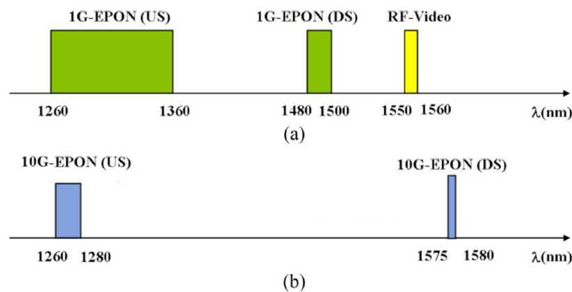
FIGURE 1.23 – Plan de longueurs d'onde de 1G-EPON et 10G-EPON [52]
