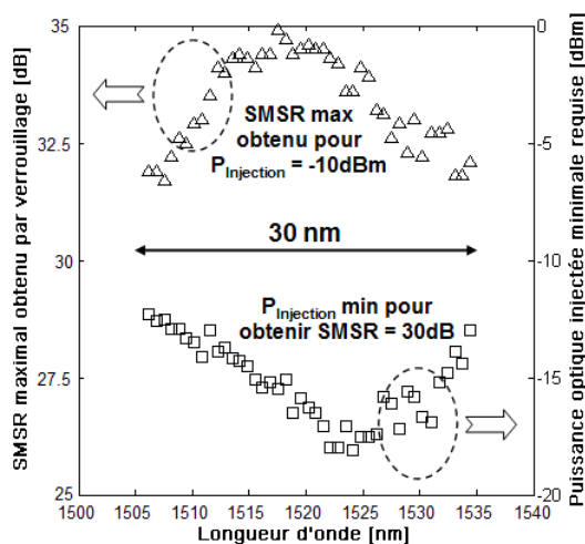
FIGURE 2.22 – Efficacité de verrouillage du laser Fabry-Perot Run1 polarisé à 40 mA [23]
