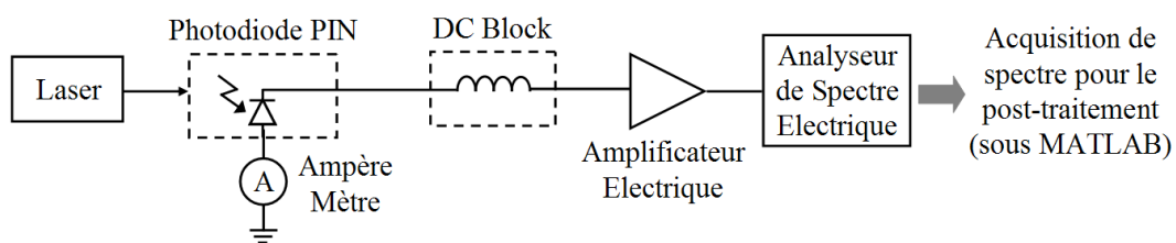
FIGURE 2.29 – Banc de mesure de RIN par la technique de détection directe
